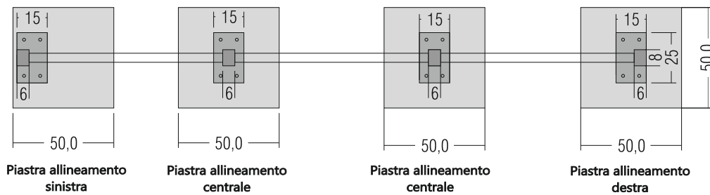
Vista dall'alto
