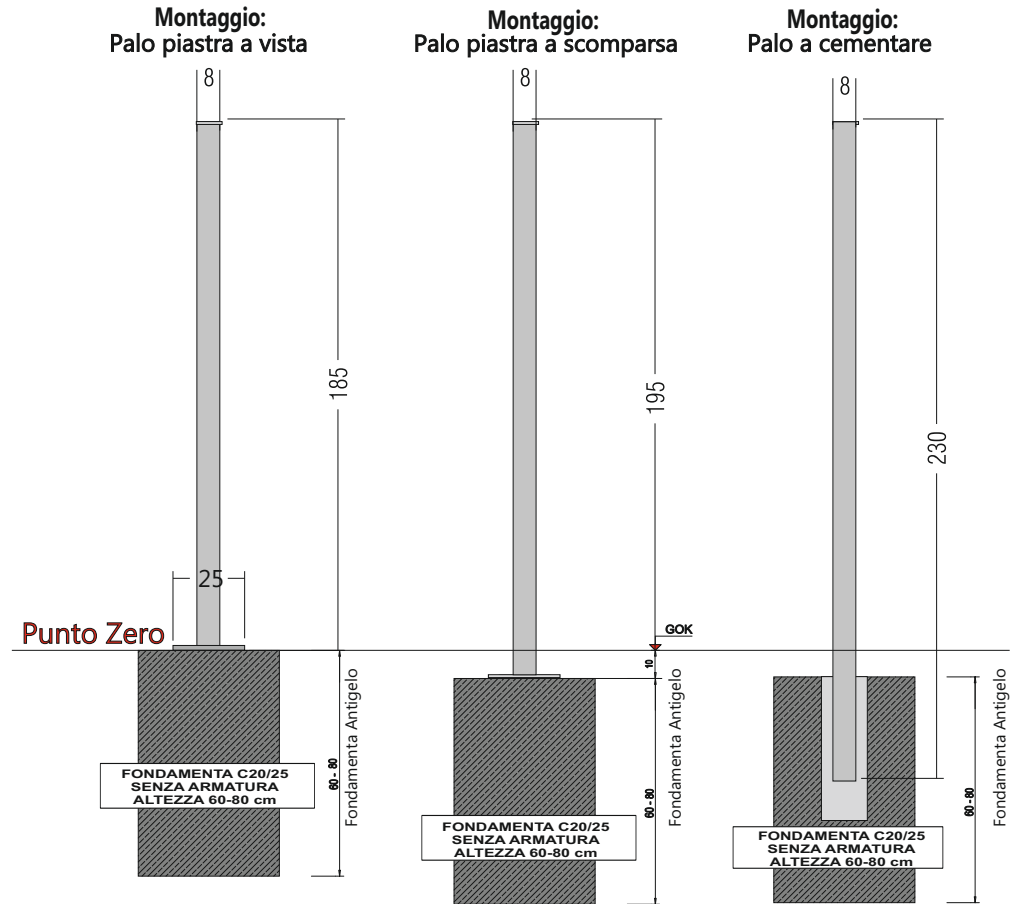
Vista laterale
